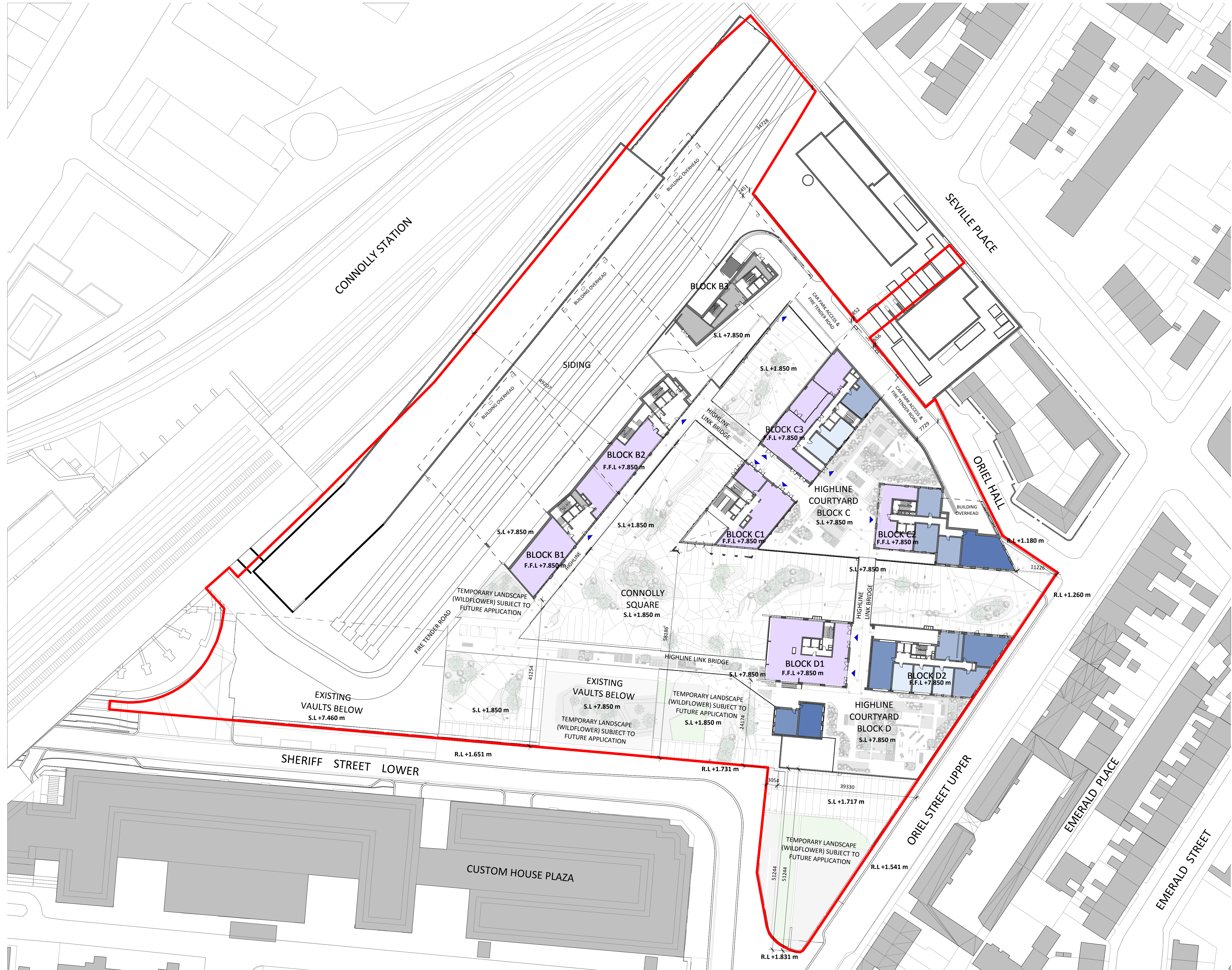
1 SITE LAYOUT PLAN - LEVEL 01 1 : 500
